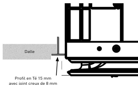
Position de montage avec faux plafond 600 x 600 mm sur profil en Té avec joint creux 8 mm
