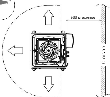
Orientation châssis pour diffusion Visual 180° uniquement
