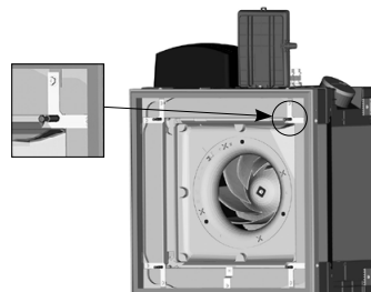
Système de fixation des diffuseurs Visual avec 4 vis imperdables
