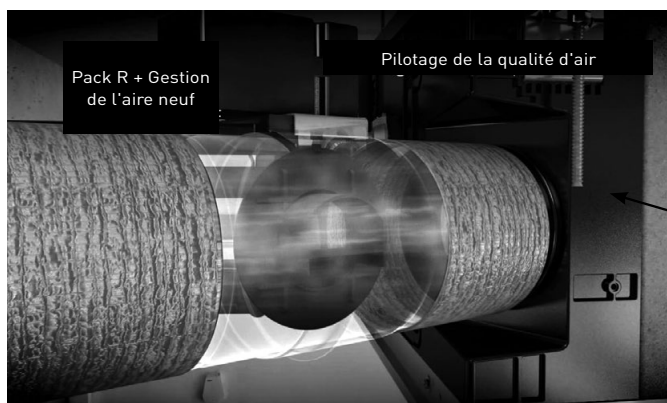
Virole Ø 100 mm, débit d'air maxi 90 m³/h préconisé. Système d'équilibrage des réseaux hors fournitures CIAT
