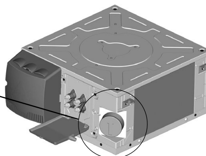
Virole Ø 100 mm, débit d'air maxi 90 m³/h préconisé. Système d'équilibrage des réseaux hors fournitures CIAT
