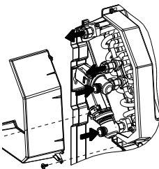
4 Leitersystem - 4-Wegeventil
