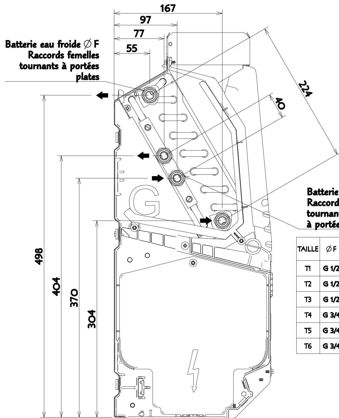
BATTERIE 4T Y (PRISES A GAUCHE)
