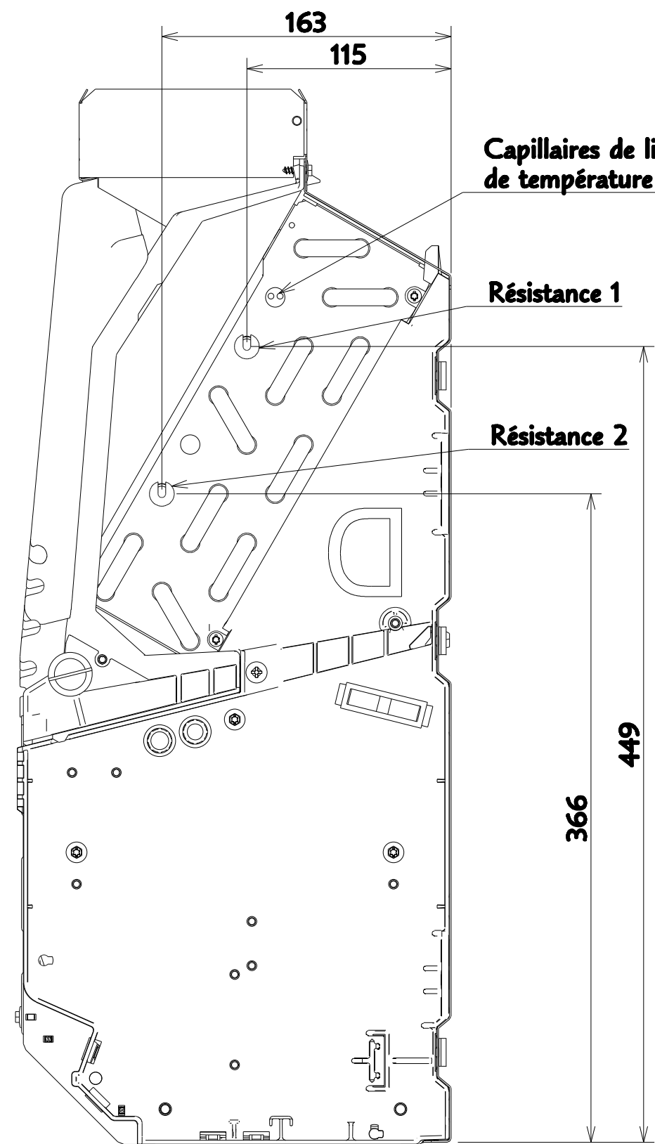
POSITION DES RESISTANCES ( PRISES A GAUCHE )
