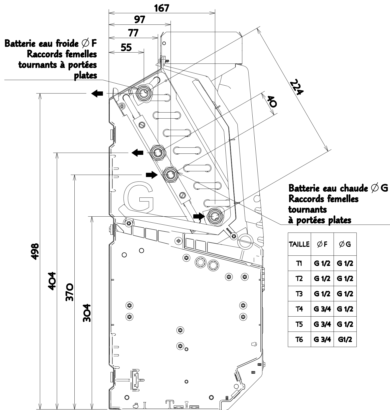
BATTERIE 4TY (PRISES A GAUCHE)
