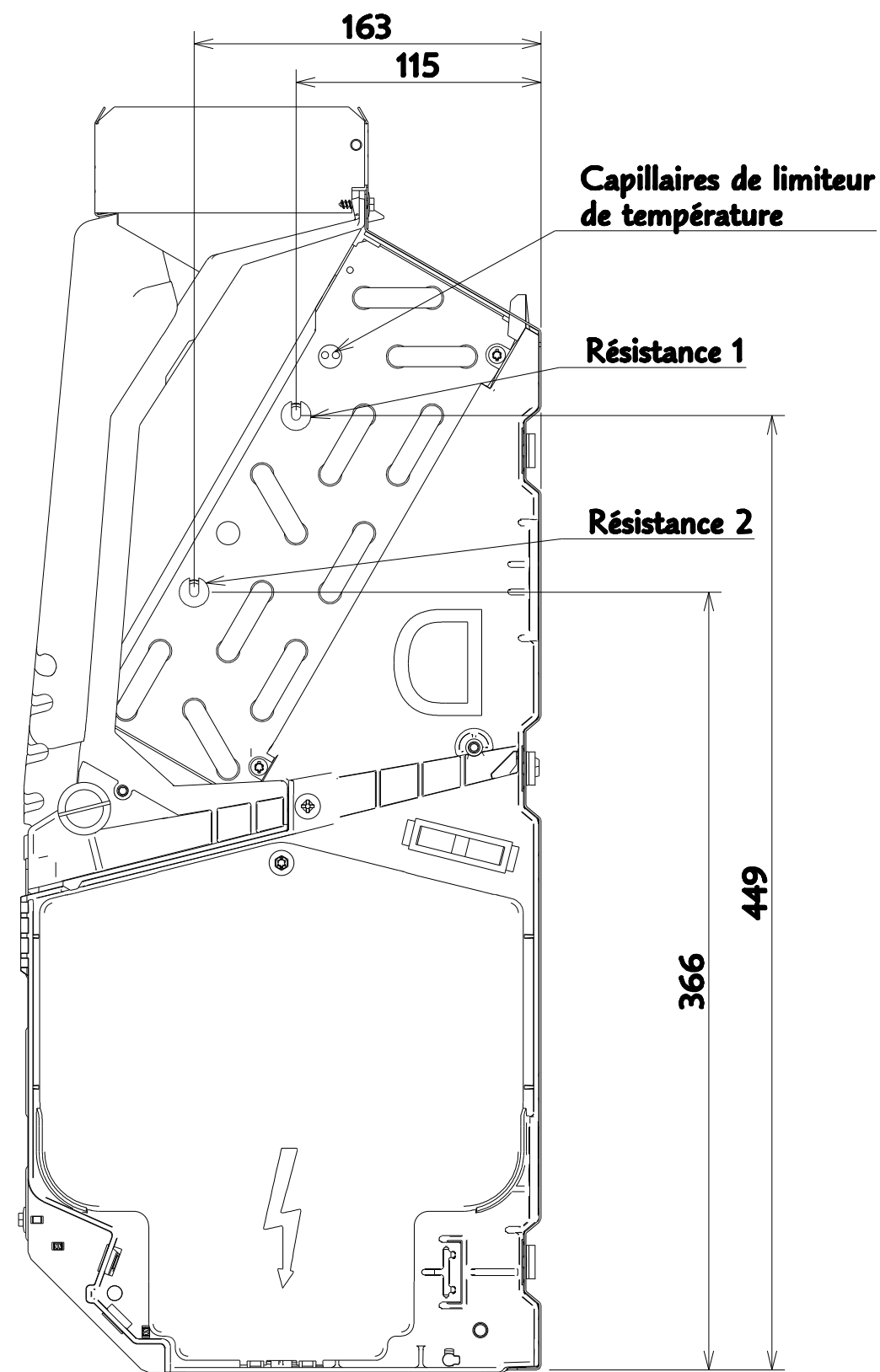
POSITION DES RESISTANCES ( PRISES A GAUCHE )
